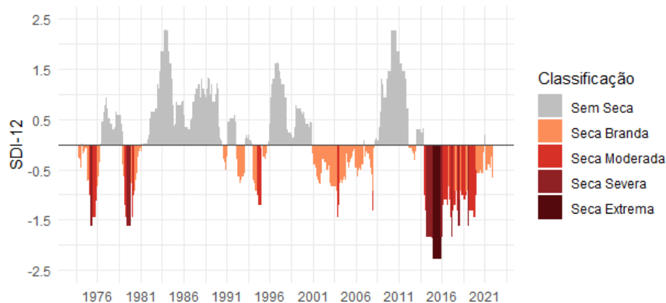
Figura 3 - Série temporal do Índice de Seca de Vazão (SDI) na escala de 12 meses.
