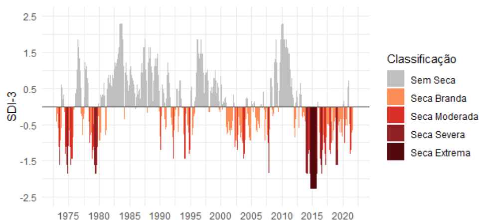
Figura 1 - Série temporal do Índice de Seca de Vazão (SDI) na escala de 3 meses.
